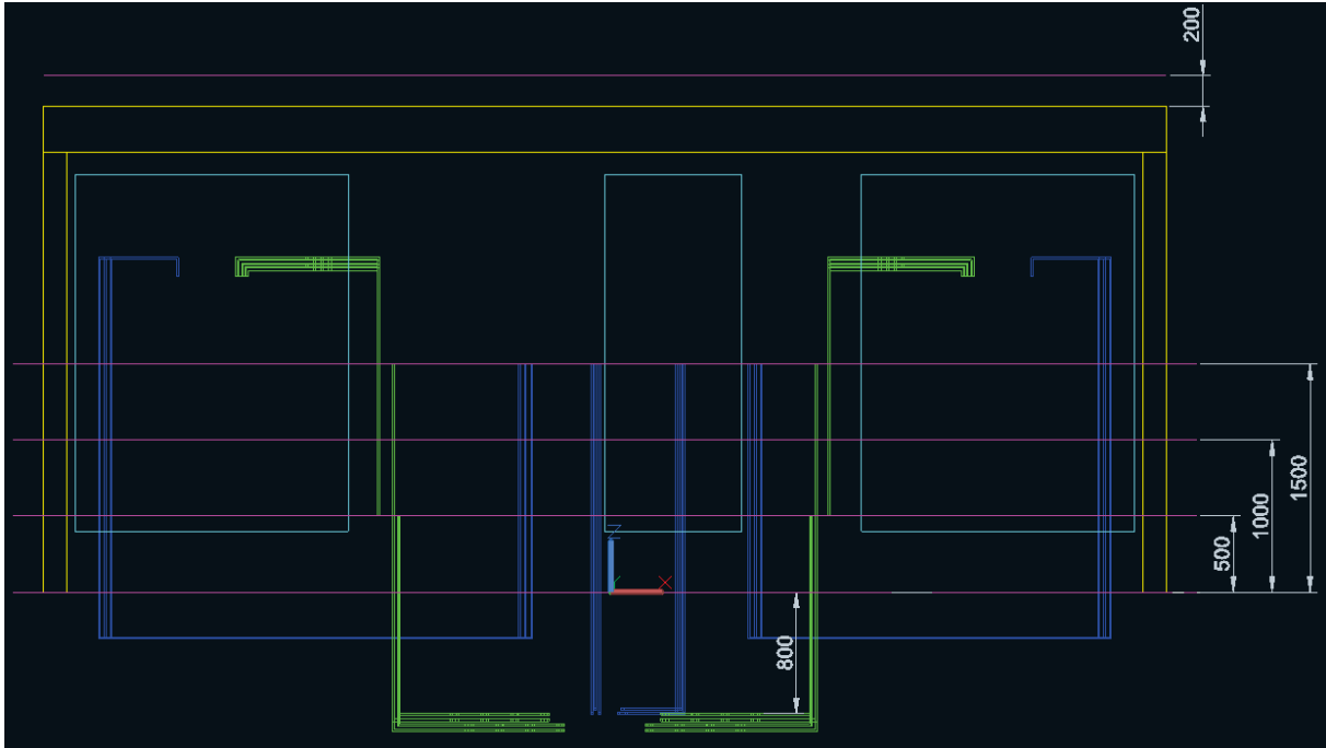
Figura 18. Vista frontal de la instalación (2L+2T) (cotas en mm).
