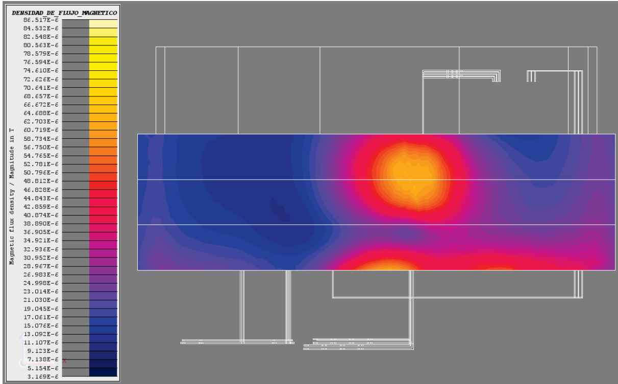
Figura 5. Densidad de flujo magnético (B[T] = Magnitud B) en el panel frontal (2L+1T [Sup]).
